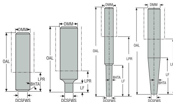
Konstrukcja 1 Konstrukcja 2 Konstrukcja 3 Konstrukcja 4
