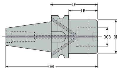
Wersja 2
