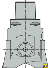
Ø 114-205 (Ø 4.488"-8.071")
