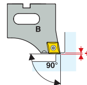
Ø 85-144 (Ø 3.346"-5.669")
